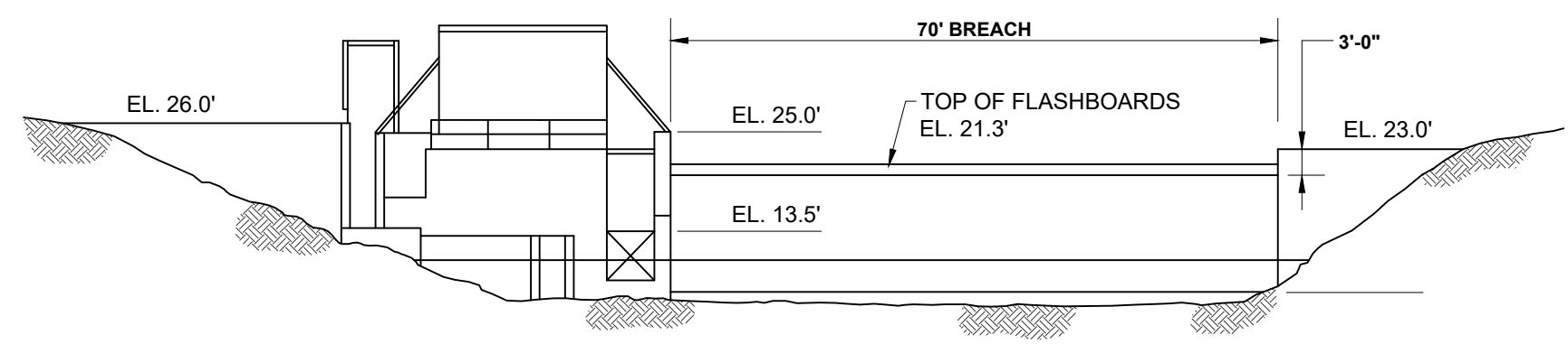
ELEVATION SCALE: 1"=20'-0"
